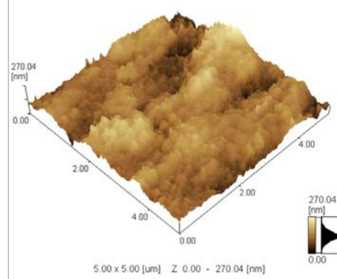
MYRA AFM Test Visual
