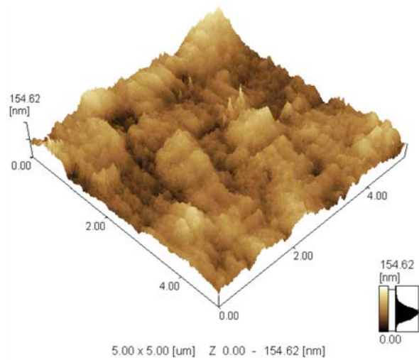
PARION AFM Test Visual
