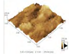
triofill AFM görüntüsü
