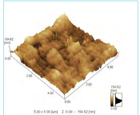
triofill + AFM görüntüsü
